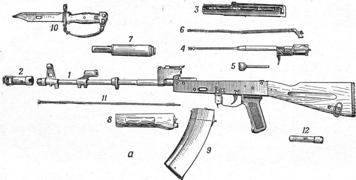
Рисунок 2 – Схема механизмов винтовки МР-512
